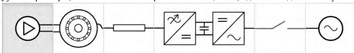
Рисунок 1. Принципиальная схема насоса
