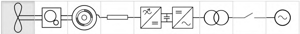
Рисунок 5. Принципиальная схема ветряной/приливной трансмиссии с тарнсформатором
