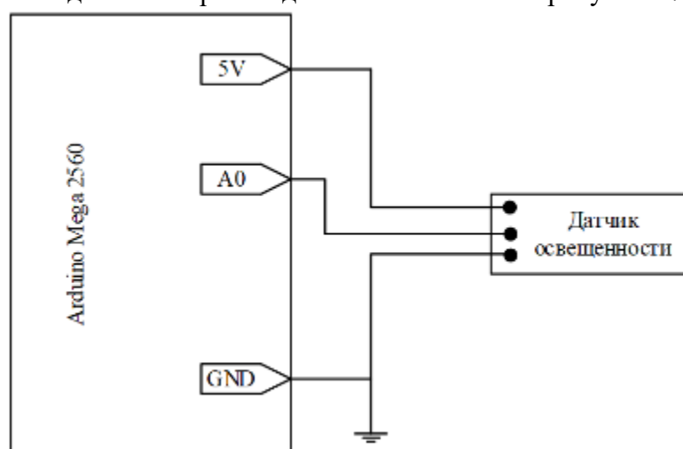
Рисунок 17 – Схема подключения датчика освещенности
