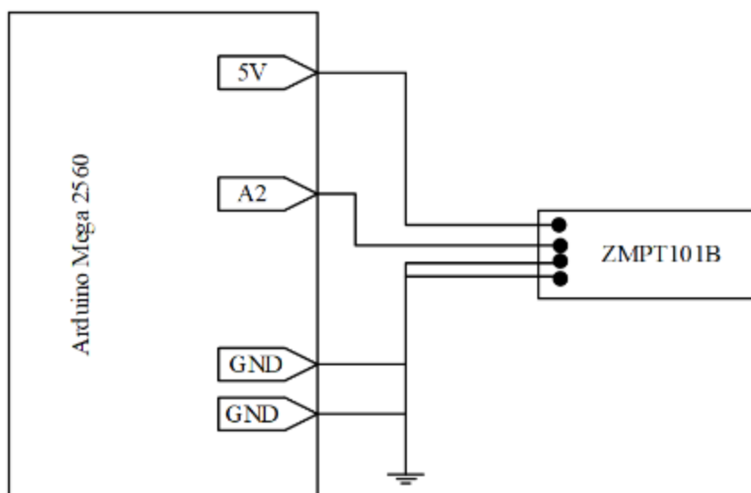
Рисунок 18 – Схема подключения датчика переменного напряжения ZMPT101B
