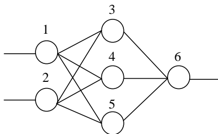
Рис. Архитектура ИНС прямого распространения
