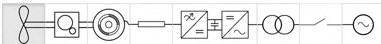
Рисунок 5. Принципиальная схема ветряной/приливной трансмиссии с тарнсформатором
