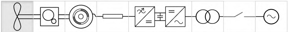
Рисунок 7. Принципиальная схема ветряной/приливной трансмиссии с тарнсформатором
