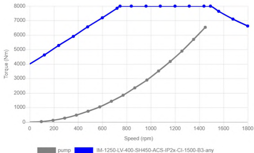
Рисунок 3. График зависимости скорости от крутящего момента
