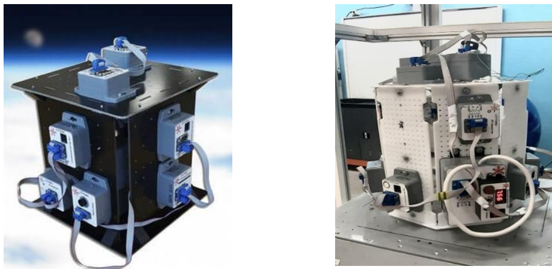
Рис. 1. Общий вид собранного конструктора «ОрбиКрафт» (или аналоги)
